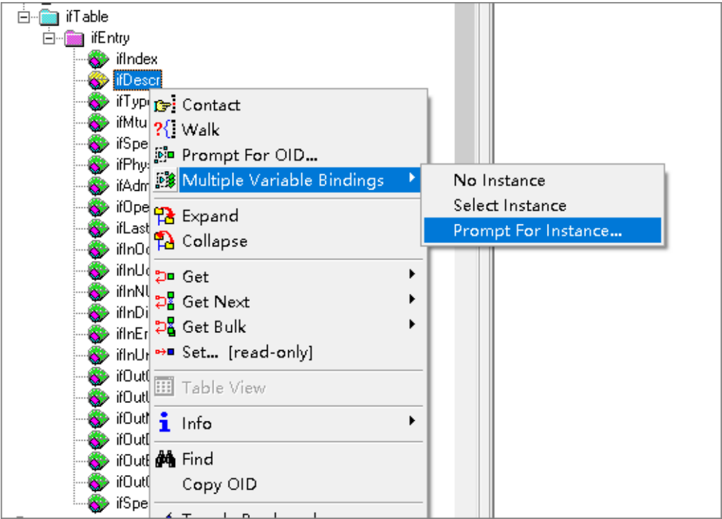
图 3-95 选择 ifDescr
