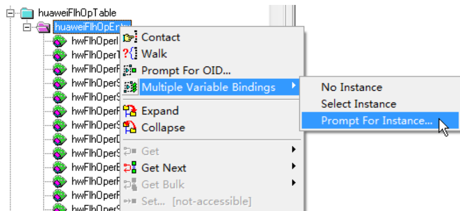
图 3-36 创建表实例
