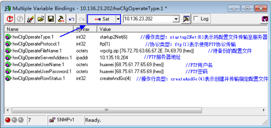
图 3-22 设置表实例
