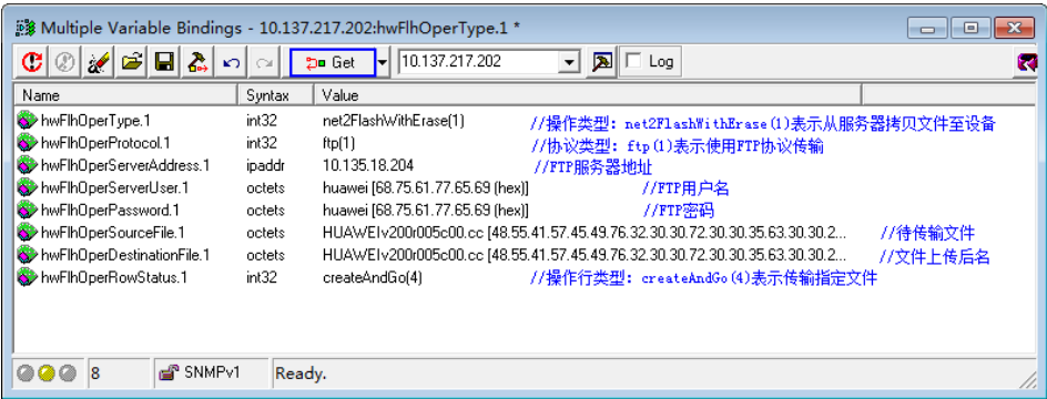
图 3-38 设置表实例
